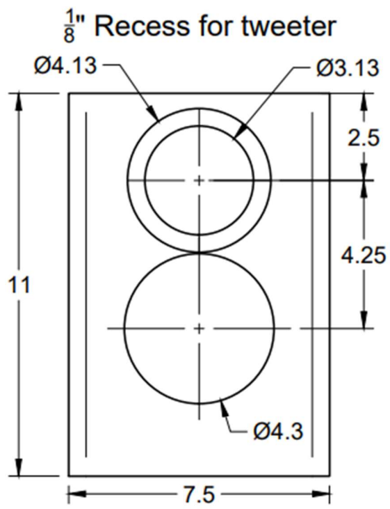
1 x Baffle
